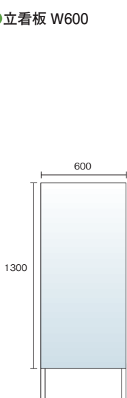
立看板 H1300
