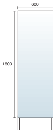
立看板 H1800
